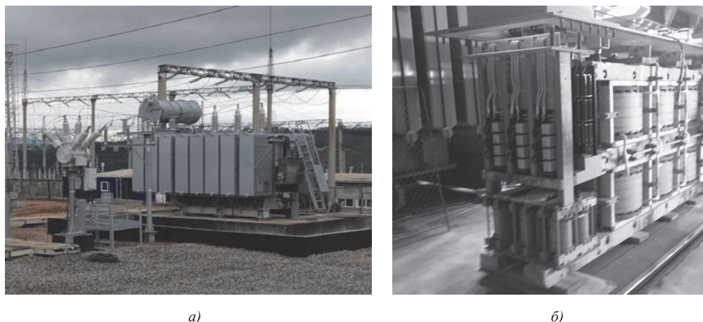
Рис. 6. УШРТм мощностью 25 МВ·А напряжением 35 кВ (полная масса 52 т, номинальные потери 200 кВт; габариты: длина 6460 мм, ширина 3565 мм, высота 4900 мм): a – общий вид; b – выемная часть
